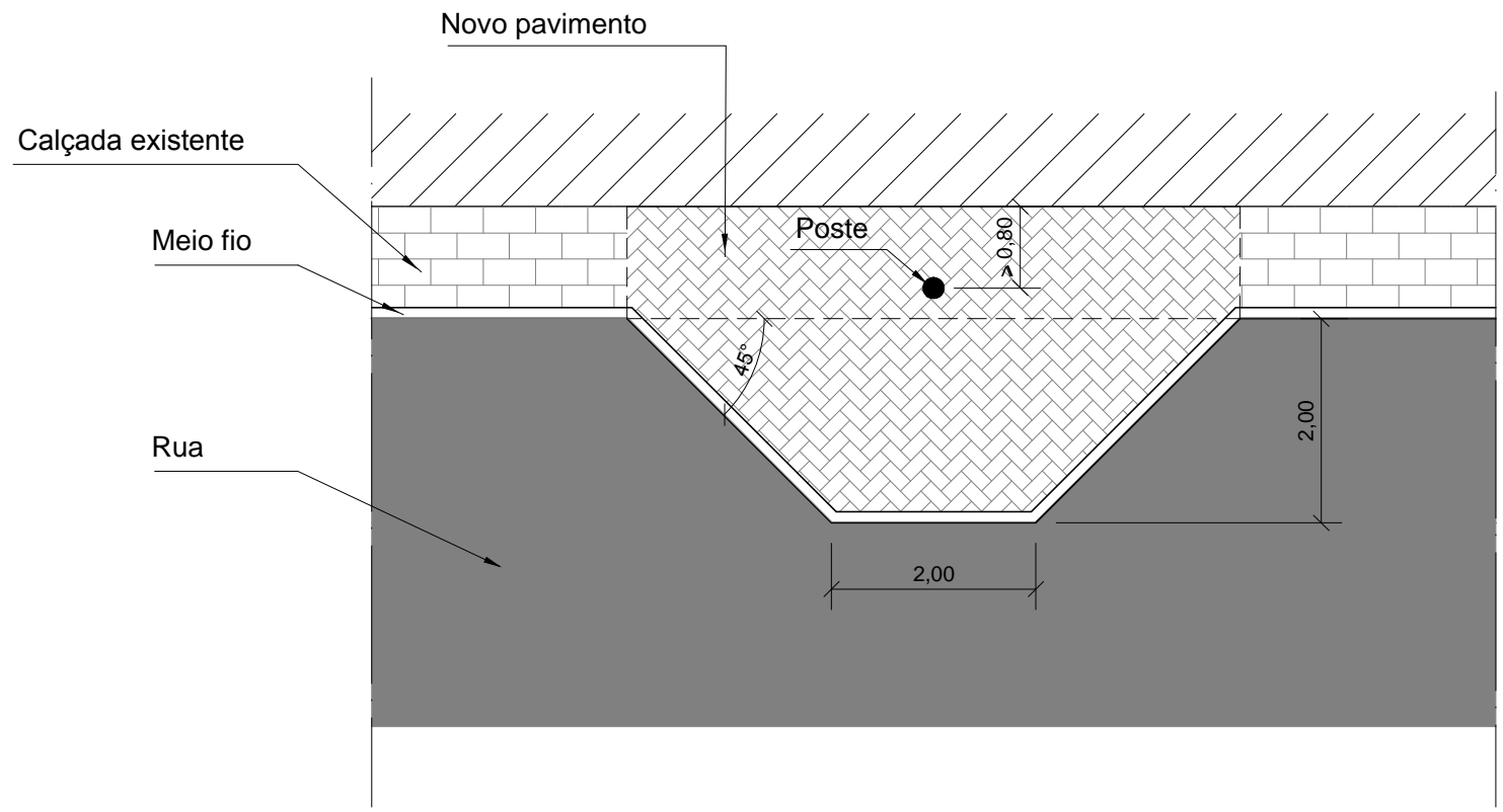
Avanço na calçada para contorno de poste ESC. 1:75
