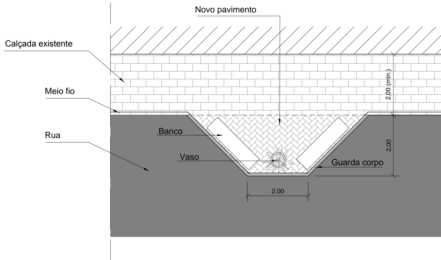
Avanço na calçada para instalação de parklet ESC. 1:75
