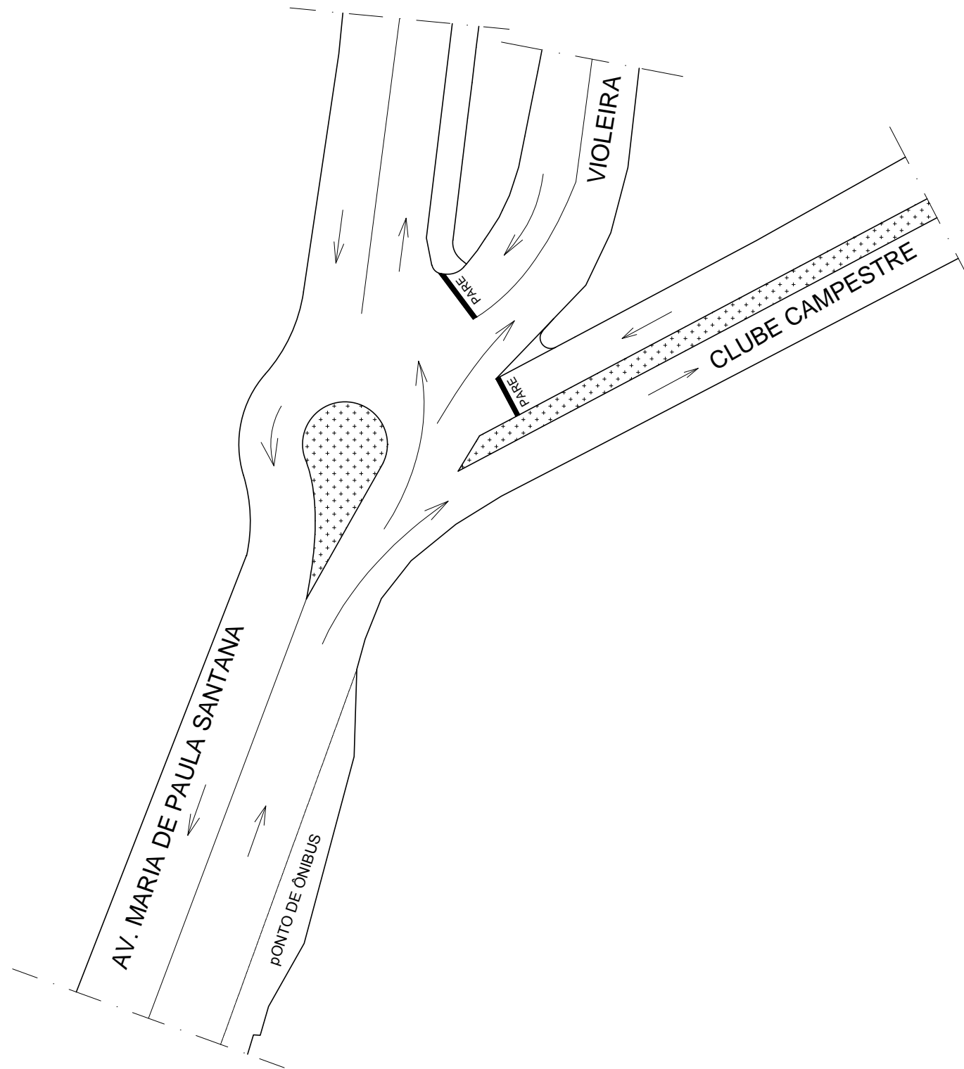
Rotatória Maria de Paula Santana x Acesso Violeira/Campestre ESC. 1:500
