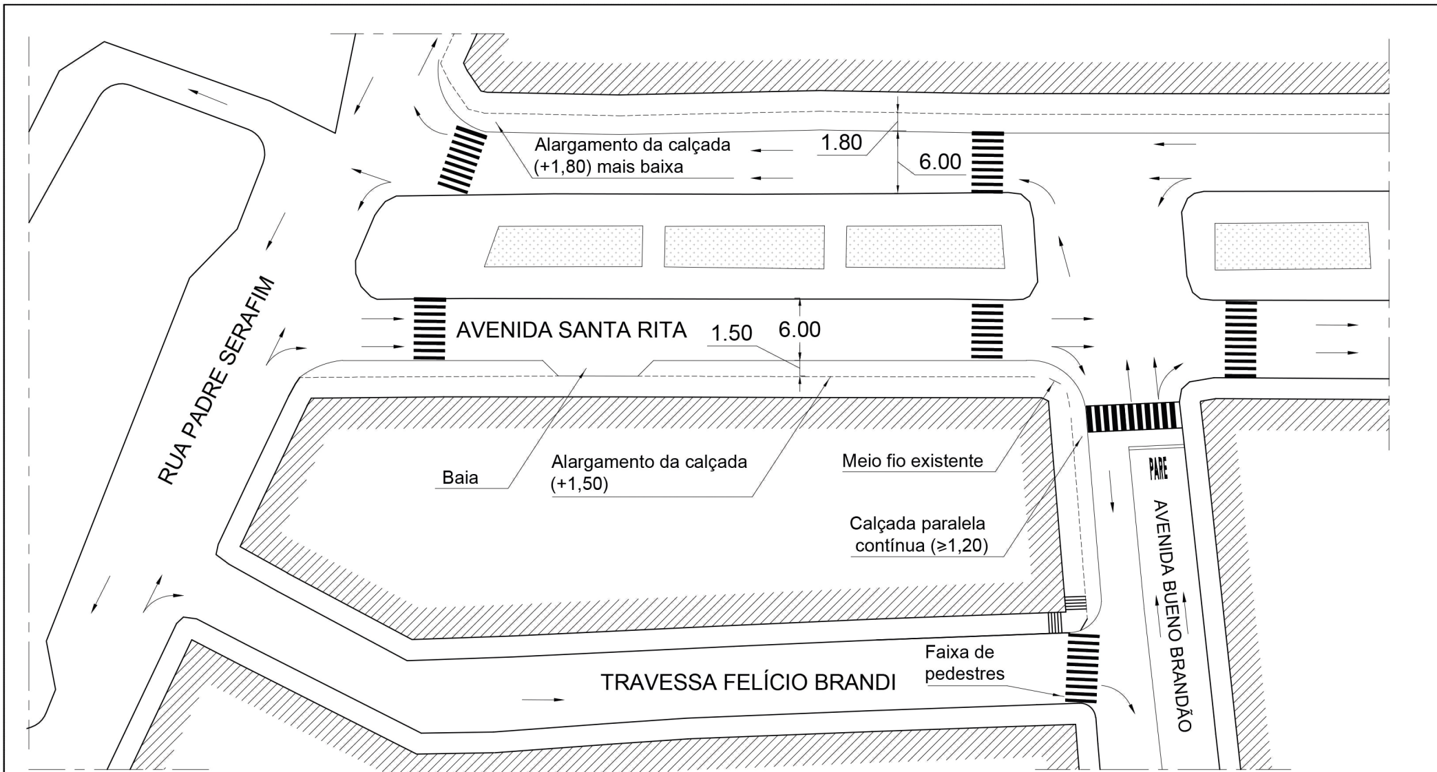
Interseção Av. Santa Rita x Av. Bueno Brandão ESC. 1:500
